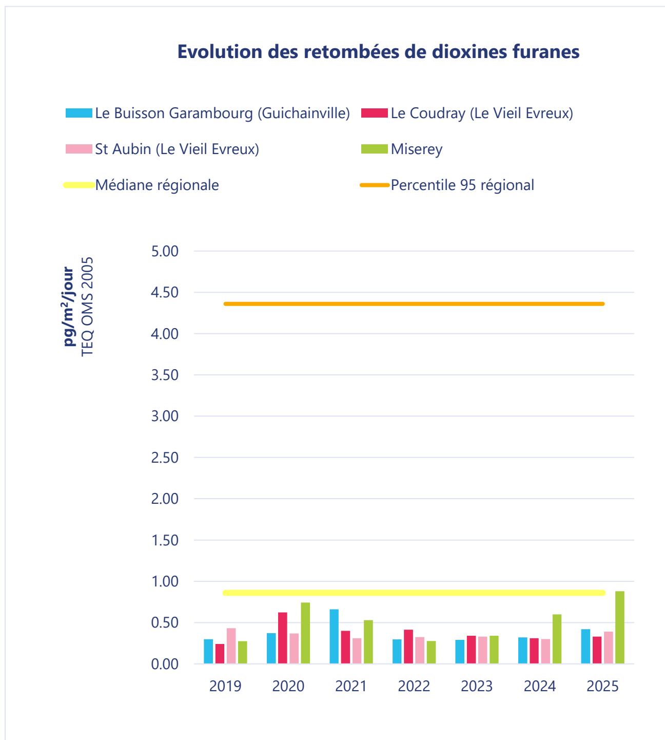
Figure 4 : Evolution des retombées de dioxines/furanes entre 2019 et 2025
