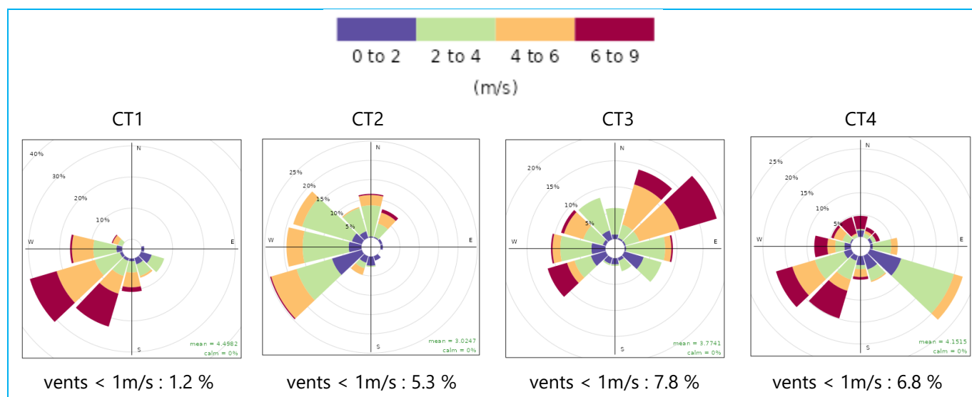
Figure 2 : Roses des vents des campagnes de mesures sur la ZI de Port-Jérôme à la station Météo Atmo Normandie de Port-Jérôme-sur-Seine.
