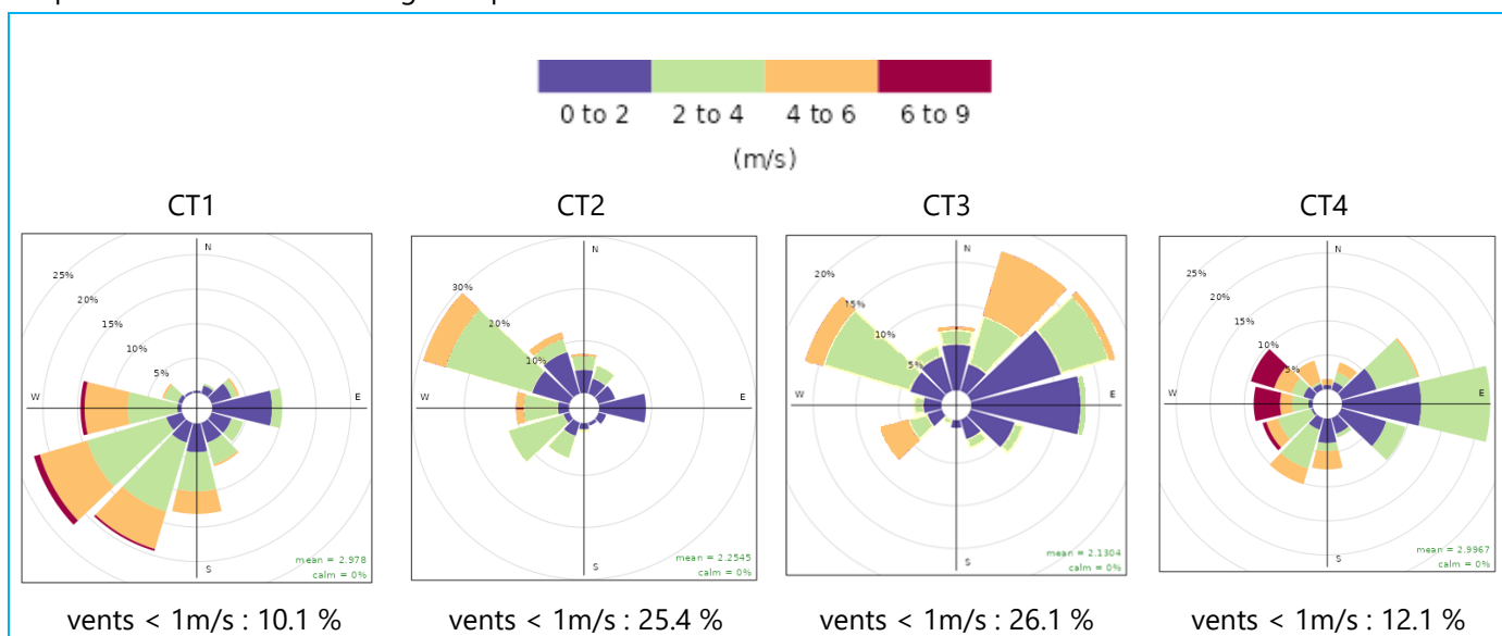
Figure 1 : Roses des vents des campagnes de mesures pour la ZI du Havre à la station Atmo Normandie Renault Sandouville.
