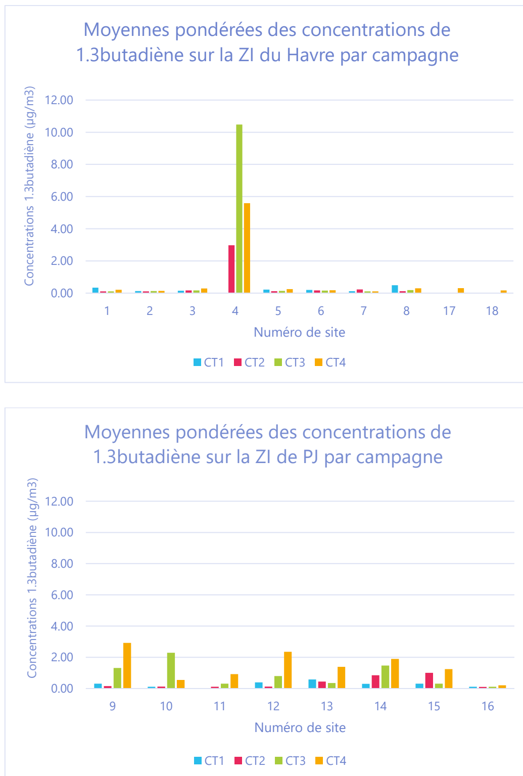
Figure 4 : Moyennes pondérées des concentrations de 1,3-butadiène par campagne pour chaque site de mesure.
