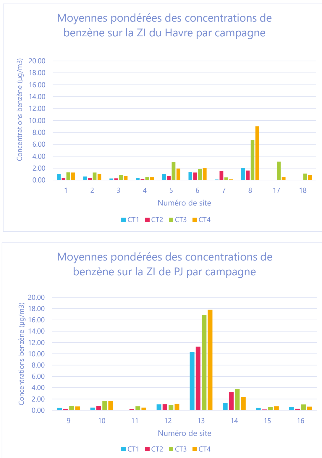
Figure 6 : Moyennes pondérées des concentrations de benzène par campagne pour chaque site de mesure.
