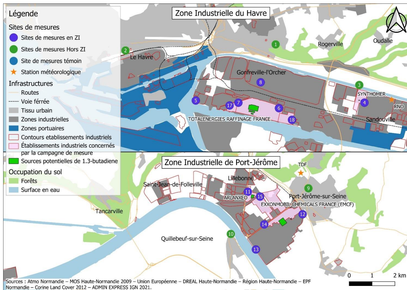
Figure 3 : Localisation des sites de mesures et des sources déclarées de 1.3-butadiène des industriels de l'étude soumis à sa surveillance.
