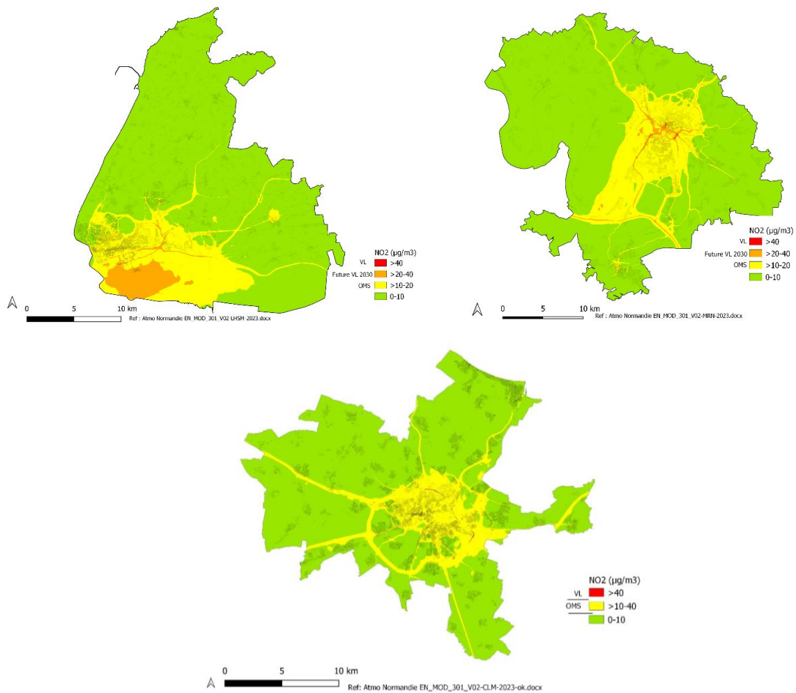
Graphique 2-4 : Cartographie de la moyenne annuelle du dioxyde d'azote (NO 2 ) en 2023 sur le périmètre LHSM (en haut à gauche), MRN (en haut à droite) et CLM (en bas)
