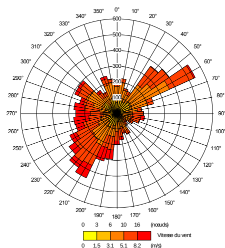
Graphique 2-7 : rose de vents utilisée pour l'étude (données 2023).
