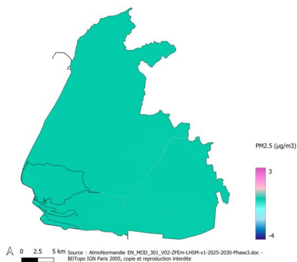
Graphique 6-28 : Cartographie des concentrations de la moyenne annuelle de PM 2.5
