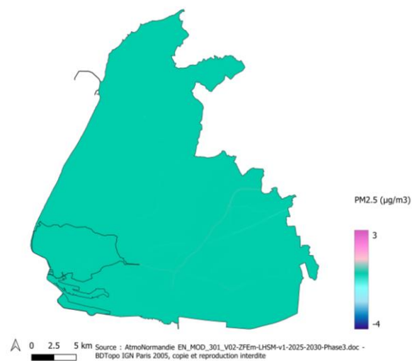
Graphique 6-14 : Cartographie des concentrations de la moyenne annuelle de PM 2.5
